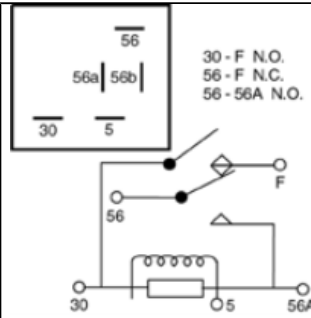
LR-35 Headlight Relay E7RY14677A; 411941583C; 111941583; 111941583A; 411941583A; 411941583B; 0332515019; 20561554; 20501766
