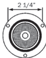
MC52 Reflex Flange
