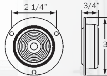
MC52 Reflex Flange
